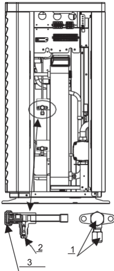
Señales de válvula de cierre: Baja presión
