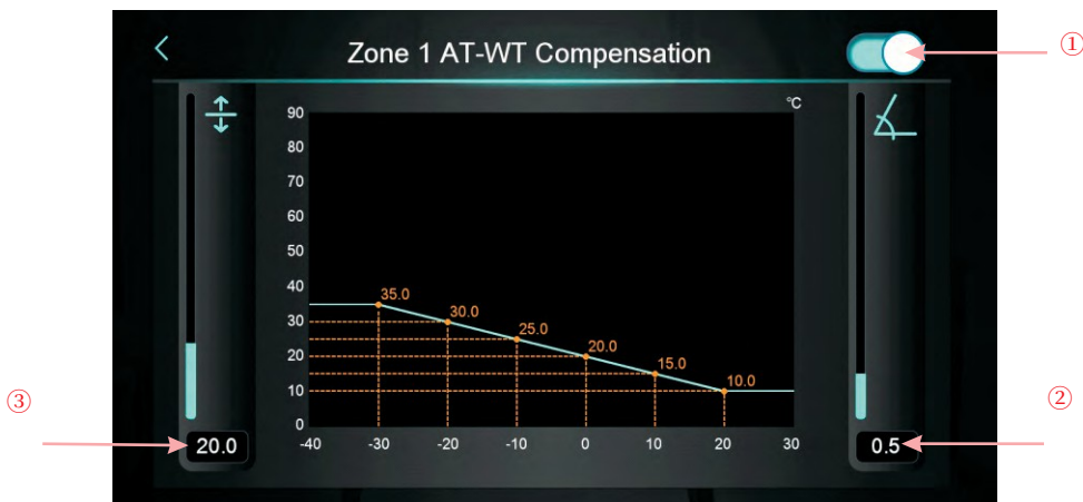
Curva de compensación meteorológica de la zona 1
