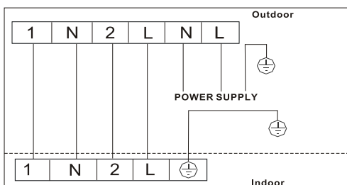
Schema di cablaggio
