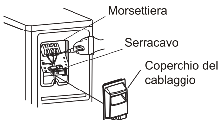
Schema di cablaggio
