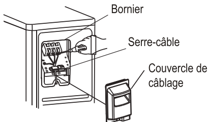
Schéma de câblage
