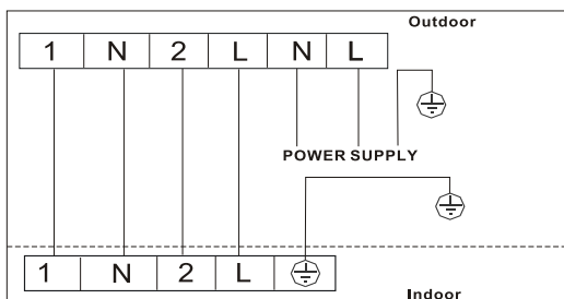
Schéma de câblage
