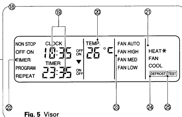
Fig. 5 Visor
