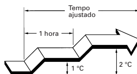
Ajustes da função paragem automática (SLEEP) em arrefecimento
