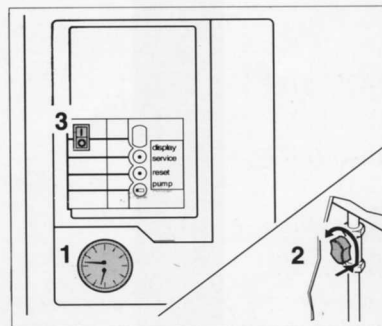
Figura 1: Pannello di comando ed indicatore di pressione
