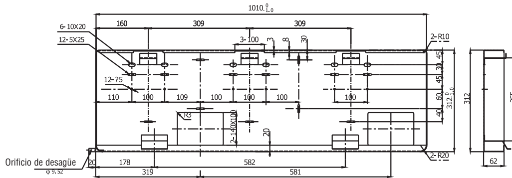
Placa de montaje de FME-12/A
