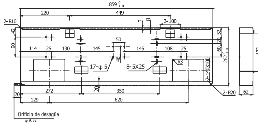
Placa de montaje de FME-12/A
