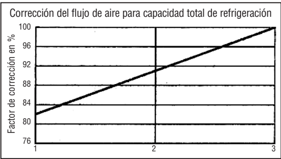
GRÁFICOS DEL FACTOR DE CORRECCIÓN DEL CAUDAL DE AIRE
