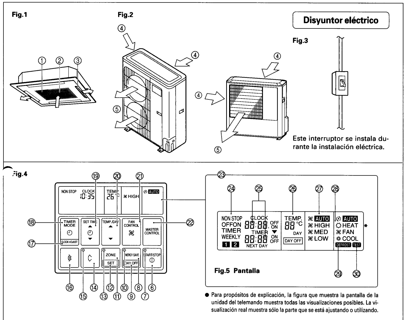
Fig.1 Unidad interior
