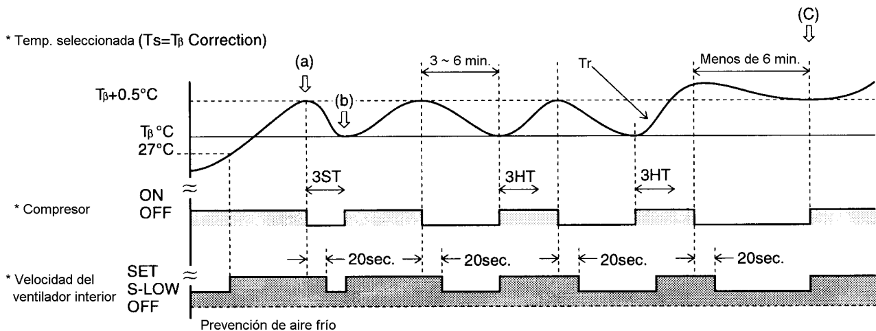
Fig. 15 Un ejemplo CONTROL DE FUNCIONAMIENTO EN CALEFACCIÓN Diagrama de flujo
