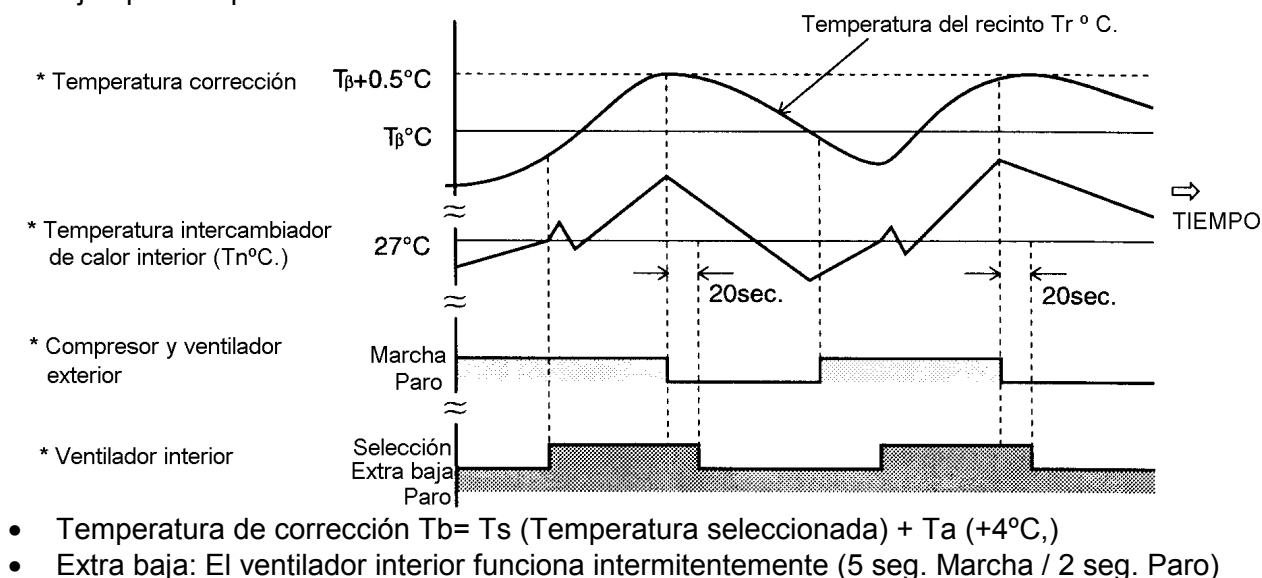
Fig. 19 Ejemplo de operación de calefacción.
