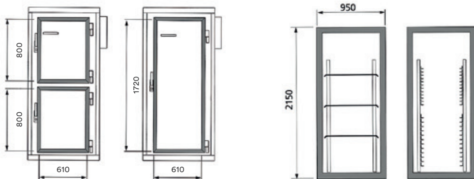
Dimensiones puertas
