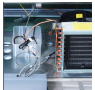
Motor extraíble para una fácil reparación.
